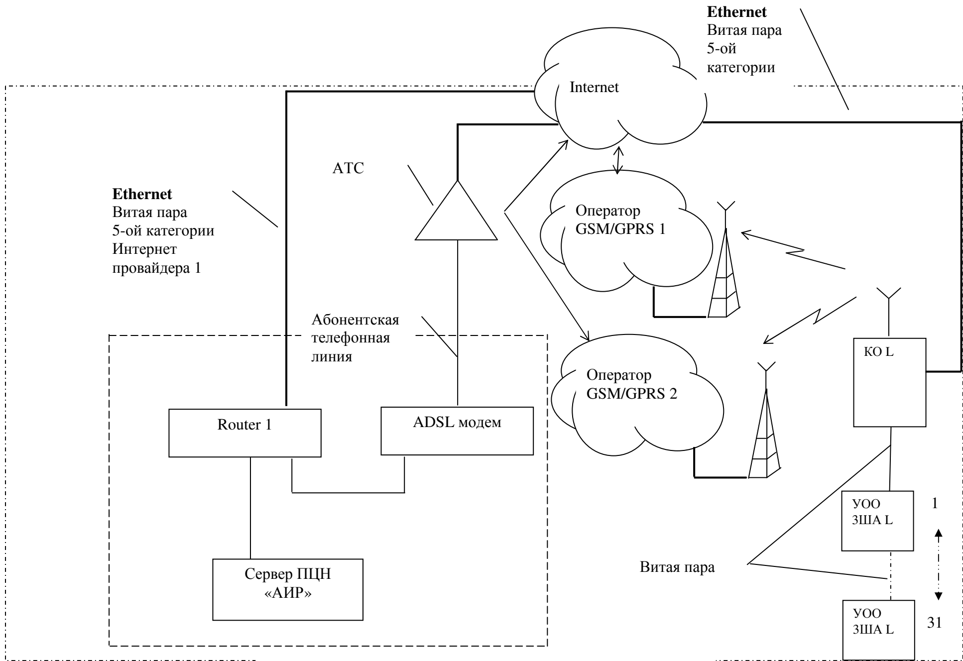
Подключение КО L и УОО ЗША L
